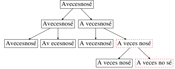
Figura 2: Ejecución del algoritmo con nivel máximo de recursión 3 y selección de un solo candidato al alcanzar resultados parciales.
