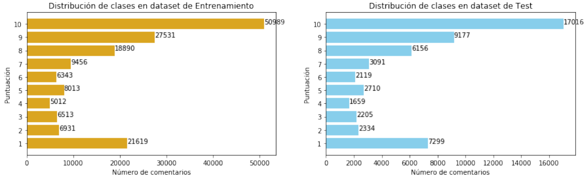
Figura 1: Distribución de las clases en los datasets de Entrenamiento y Test
