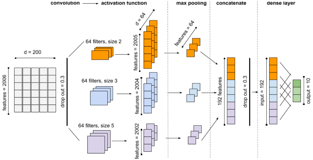
Figura 2: Arquitectura de nuestro sistema
